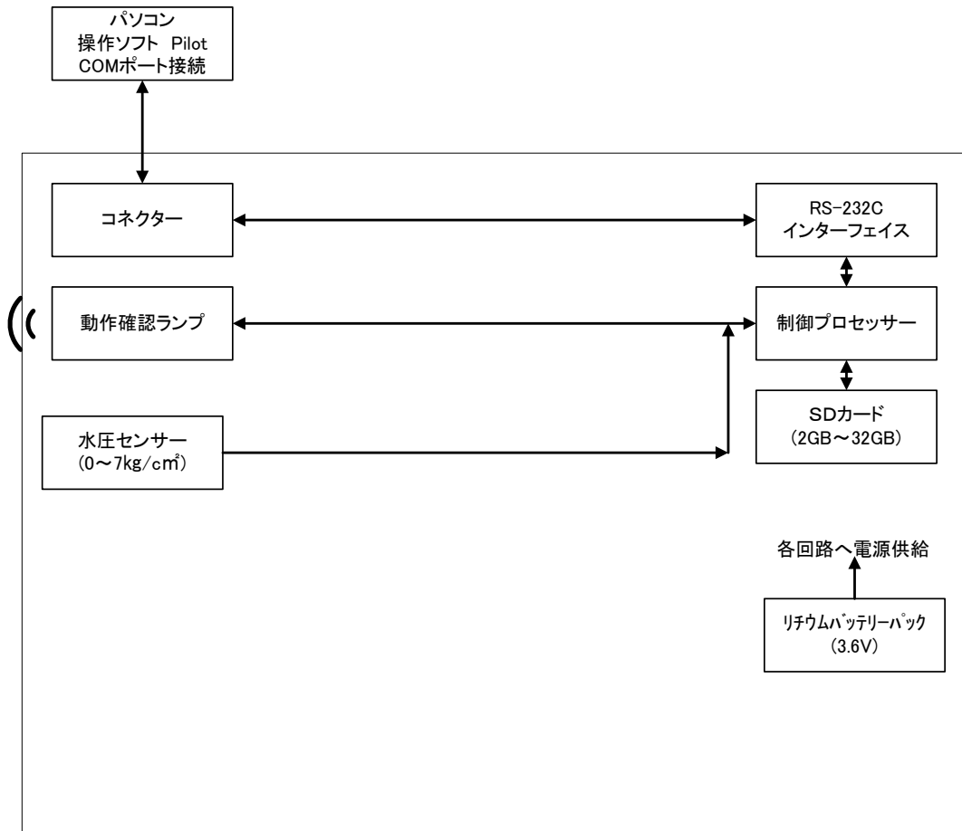
図1-2 ブロック図
